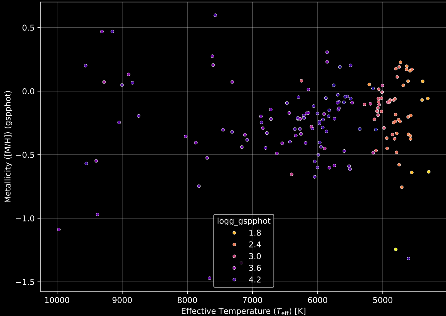
GALAH DR4 Field: [3702] Stellar Population Parameters (n= 161)
